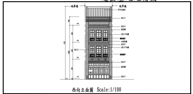
建築物立面圖
