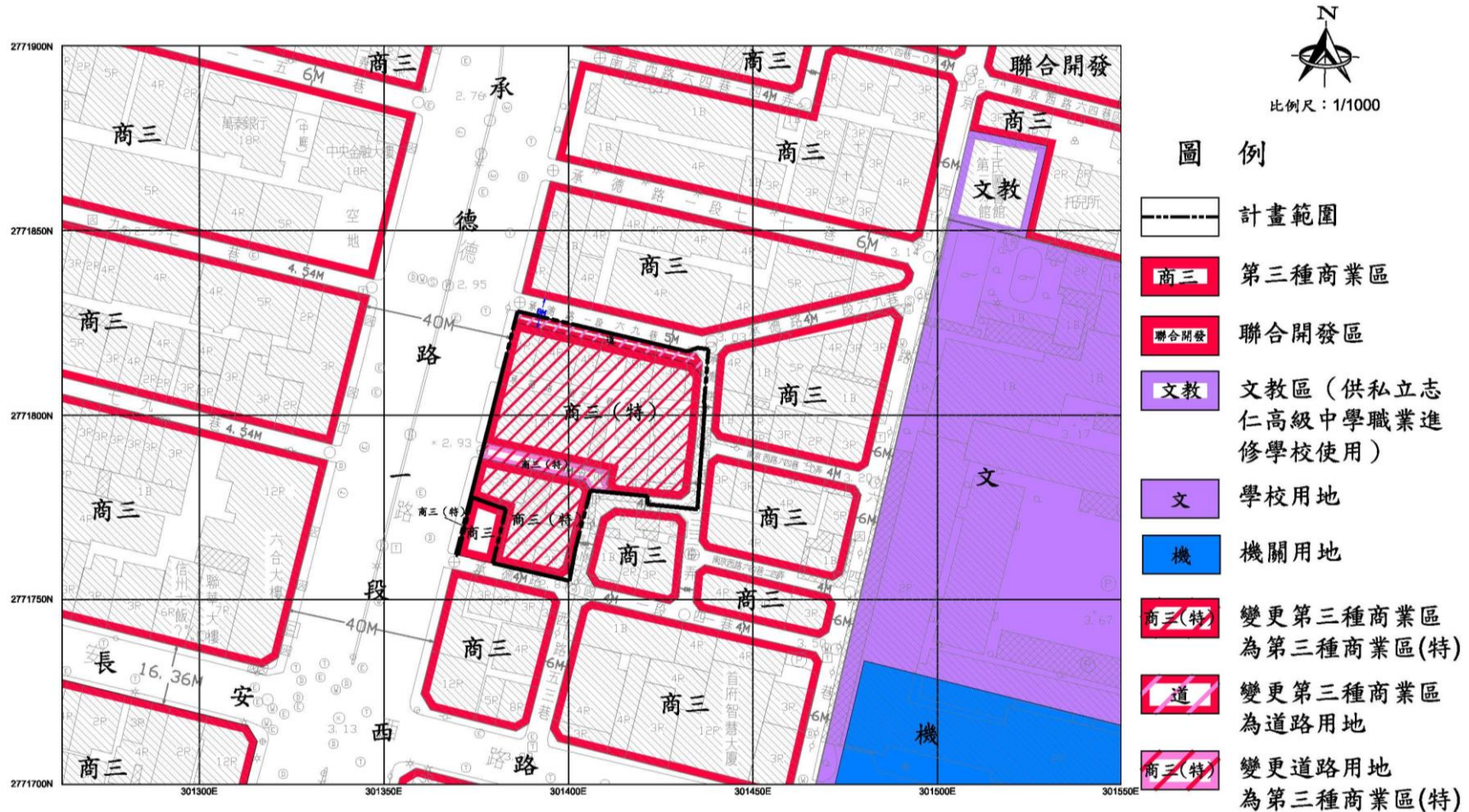
變更臺北市大同區市府段一小段 288-4 地號等第三種商業區、道路用地為道路用地、第三種商業區（特）細部計畫案示意圖
